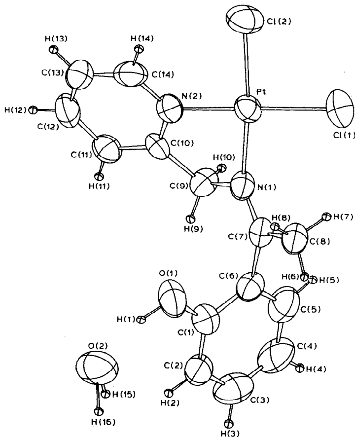
Fig. 1. Structure moléculaire du complexe VIib.
